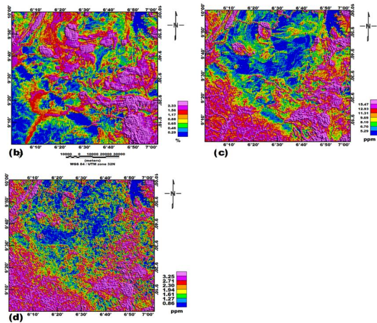
Figure 3: Airborne radiometric anomaly maps of the study area (b) Potassium (c) Thorium (d) Uranium
